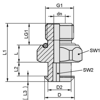
Datos de diseño SC 050 G1/4-AG SW410
