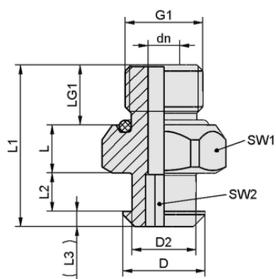
Конструктивные данные SC 040 M5-AG
