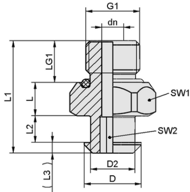
Tasarım verileri SC 040 M5-AG
