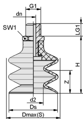
デザインデータ FSG 5 NBR-ESD-55 M5-AG
