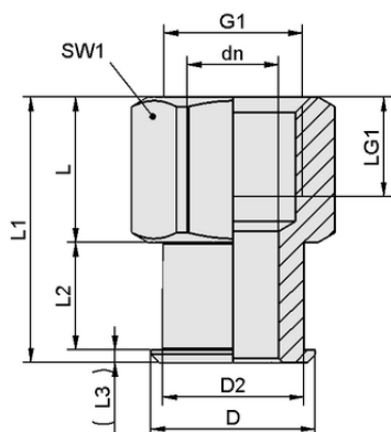
Dati di costruzione SC 050 G1/8-IG
