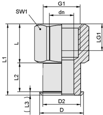
Tasarım verileri SC 030 G1/8-IG
