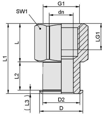
Tasarım verileri SC 020 M5-IG
