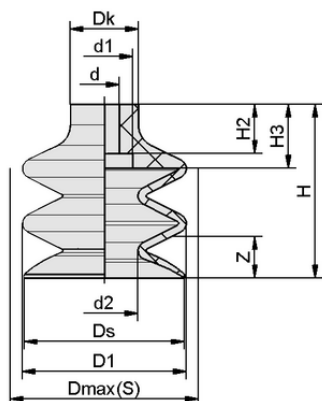
Конструктивные данные FG 42 SI-MD-55 N018
