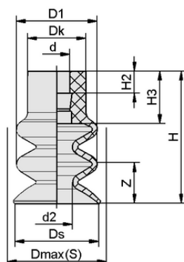
Конструктивные данные FG 12 NBR-ESD-55 N062
