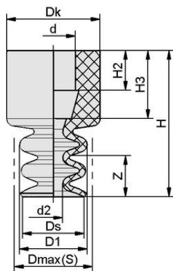
Datos de diseño FG 9 NBR-ESD-55 N062
