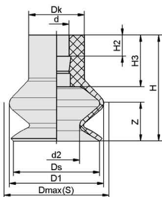
Données de construction FGA 20 NBR-ESD-55 N062
