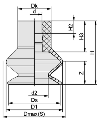
Datos de diseño FGA 20 NBR-ESD-55 N062
