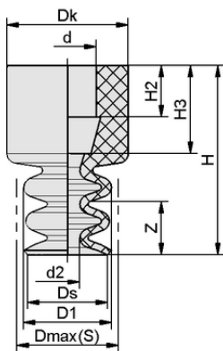
Datos de diseño FG 9 SI-MD-55 N016
