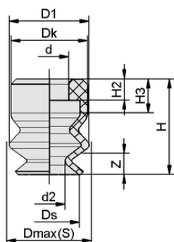
デザインデータ FGA 2 NBR-55 N003
