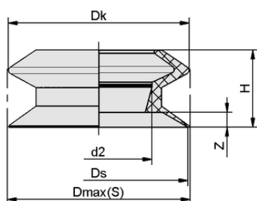
Конструктивные данные FLSA 30 NBR-ESD-55
