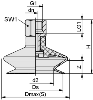
Tasarım verileri FSGA 33 SI-MD-55 G1/4-IG
