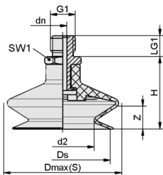
デザインデータ FSGA 33 SI-MD-55 G1/4-AG
