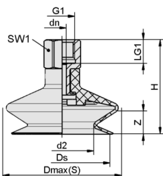
Datos de diseño FSGA 25 SI-MD-55 G1/8-IG
