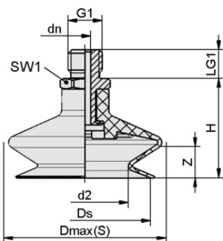
Datos de diseño FSGA 25 SI-MD-55 G1/8-AG
