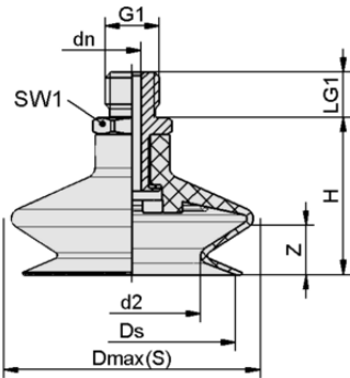
Tasarım verileri FSGA 25 SI-MD-55 G1/8-AG
