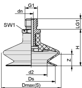
Конструктивные данные FSGA 25 SI-MD-55 G1/8-AG
