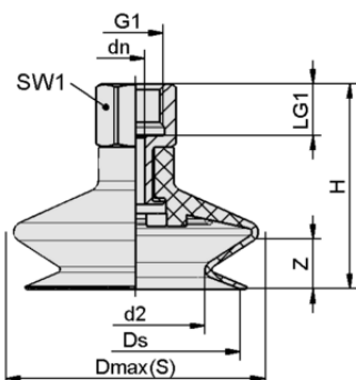
Datos de diseño FSGA 22 SI-MD-55 G1/8-IG
