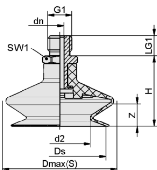
Dati di costruzione FSGA 22 SI-MD-55 G1/8-AG
