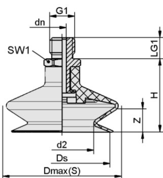
Конструктивные данные FSGA 22 SI-MD-55 G1/8-AG
