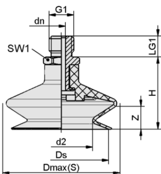
Dati di costruzione FSGA 20 SI-MD-55 G1/8-AG
