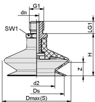
デザインデータ FSGA 20 SI-MD-55 G1/8-AG
