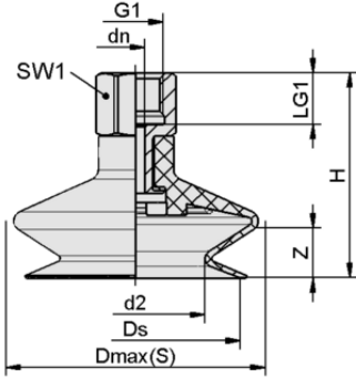
Tasarım verileri FSGA 14 SI-MD-55 G1/8-IG
