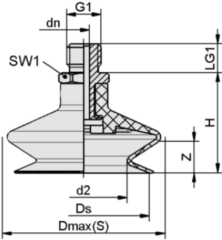
Tasarım verileri FSGA 14 SI-MD-55 M5-AG
