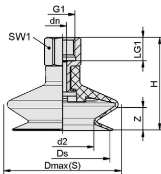
デザインデータ FSGA 25 SI-HD-65 G1/8-IG
