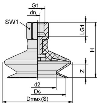
デザインデータ FSGA 11 SI-HD-65 G1/8-IG
