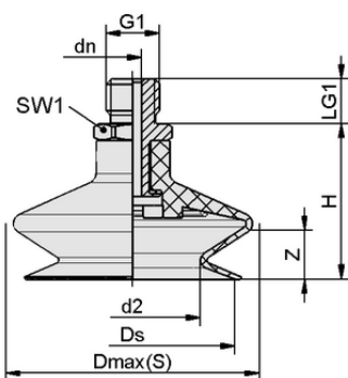
デザインデータ FSGA 11 SI-HD-65 G1/8-AG
