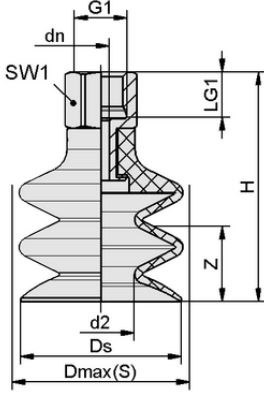
Tasarım verileri FSG 14 SI-HD-65 G1/8-IG
