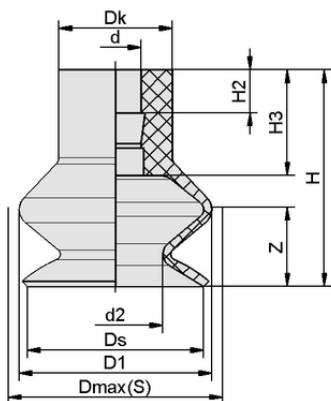
Données de construction FGA 20 SI-HD-65 N016
