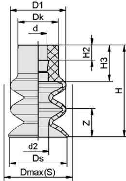
Tasarım verileri FG 18 SI-HD-65 N016
