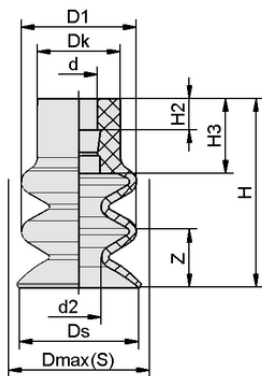
Données de construction FG 18 SI-HD-65 N016
