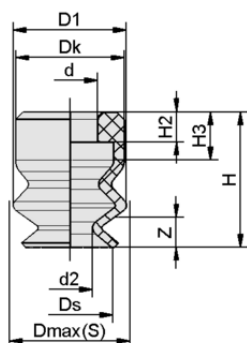
デザインデータ FGA 4 HT1-60 N003
