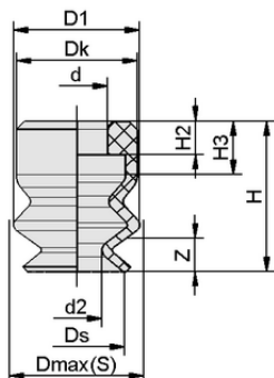
デザインデータ FGA 4 NBR-55 N003
