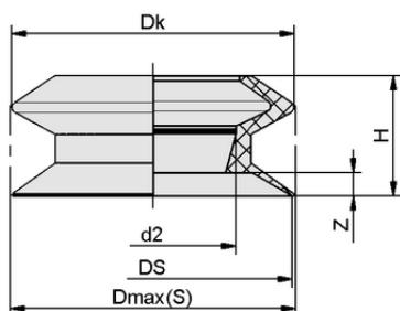
デザインデータ FLSA 50 SI-MD-55
