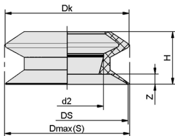
Konstruktionsdaten FLSA 50 SI-MD-55
