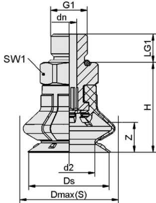
Tasarım verileri SPB1 80 ED-65 G1/2-AG
