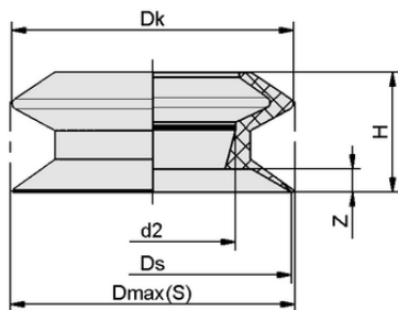
Datos de diseño FLSA 20 SI-HD-65
