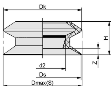
Конструктивные данные FLSA 40 SI-HD-65
