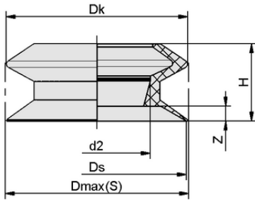
Tasarım verileri FLSA 40 SI-HD-65
