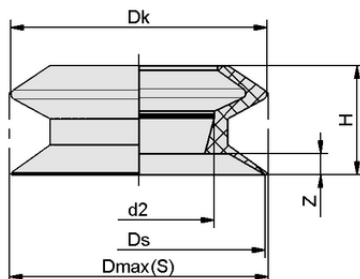
デザインデータ FLSA 40 SI-HD-65
