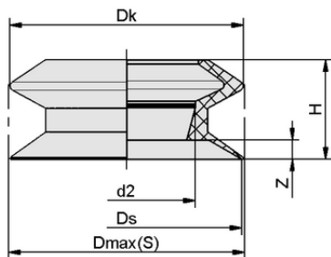
Konstruktionsdaten FLSA 30 SI-HD-65
