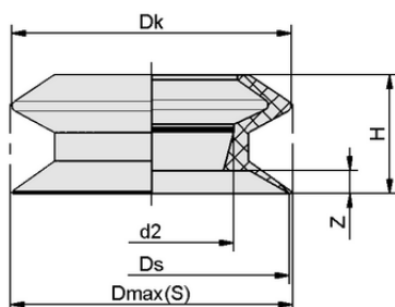
Données de construction FLSA 30 SI-HD-65
