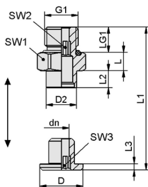
Datos de diseño SC 050-AR G1/4-AG MOD
