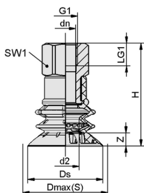
Конструктивные данные SPB2f 30 SI-55 G3/8-IG
