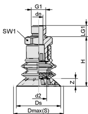
Конструктивные данные SPB2f 30 SI-55 G3/8-AG
