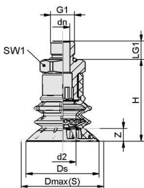
Конструктивные данные SPB2f 30 SI-55 G1/8-AG
